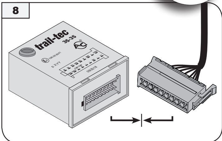
Modul Trail-tec 35-35 → Stecker 18 pin E-Satz modul Trail-tec 35-35 → socket 18 pin e-kit
