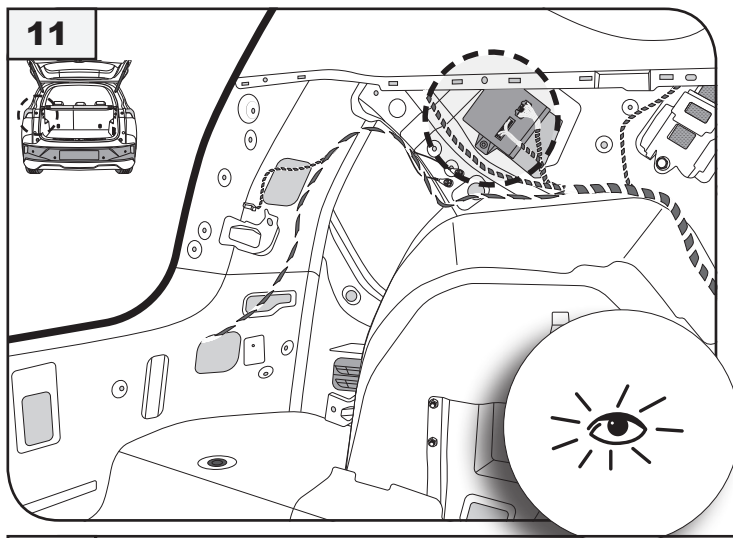
Fahrzeuge Stecker wh 24 pin car socket wh 24 pin
