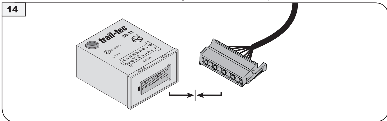
Modul Trail-tec 35-31 → Stecker 18 pin E-Satz modul Trail-tec 35-31 → socket 18 pin e-kit
