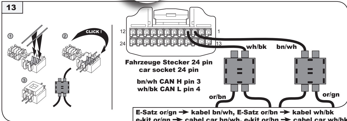
Fahrzeuge Stecker wh 24 pin car socket wh 24 pin
