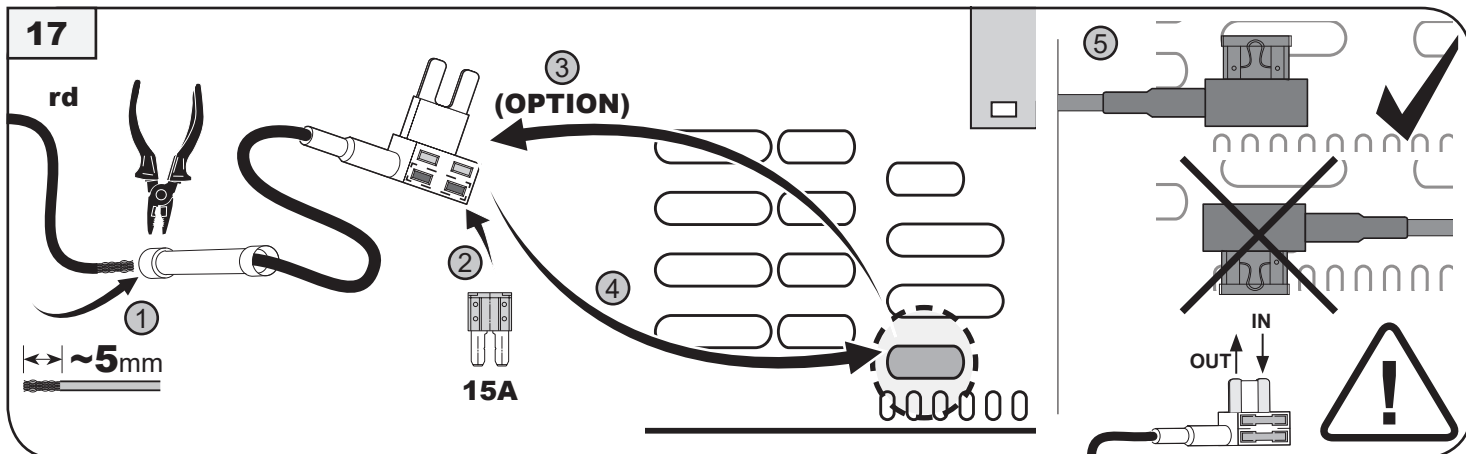
Sicherung 15A → E-Satz rd → Sicherungskasten F24 fuse 15A → e-kit rd → fusebox F24
