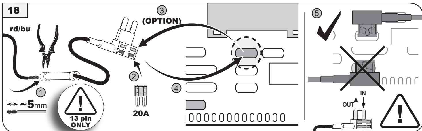
Sicherung 20A → E-Satz rd/bu → Sicherungskasten F05 fuse 20A → e-kit rd/bu → fusebox F05
